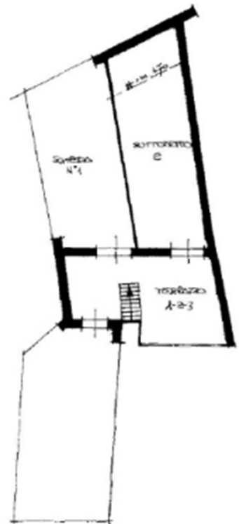
PIANO 3° (SOTTOTETTO) H MEDIA 2,60
